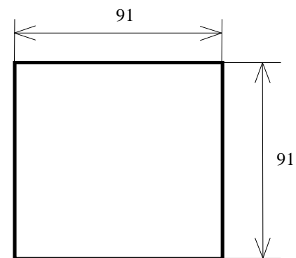
Рис.1. Вырез в щите для крепления контроллера.
