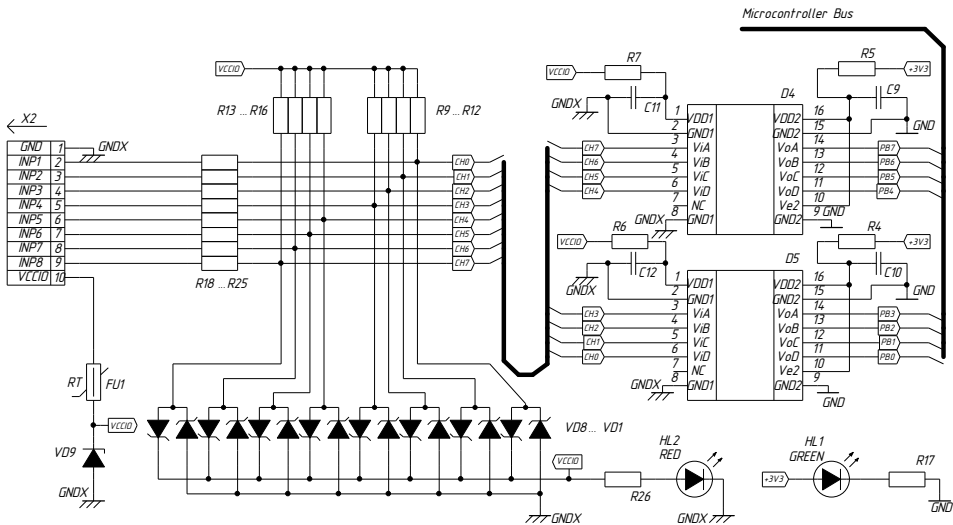
Электрическая принципиальная схема входных цепей прибора "LOGIC-U ISL"
