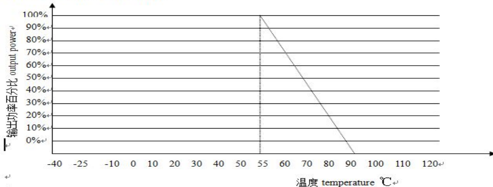
工作环境温度与负载特性
